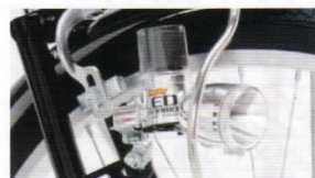
LED軽ダイナモ 高輝度LEDライト 軽く静かなダイナモローラー
